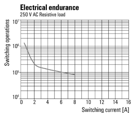
Trwałość elementów elektrycznych 250 V AC obciążenie rezystancyjne
