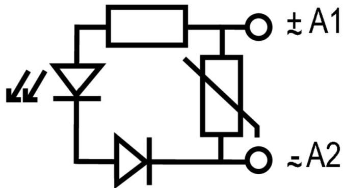
Schemat połączeń
