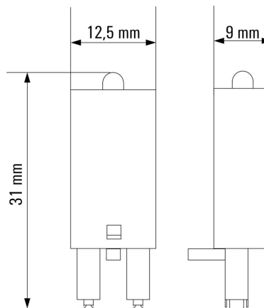
Rysunek wymiarowany
