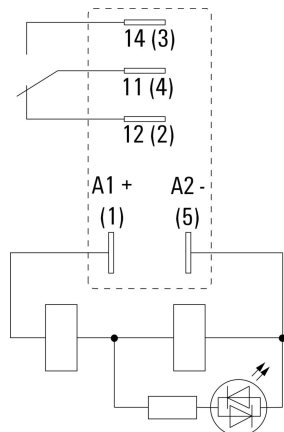
Widok kołków od spodu
