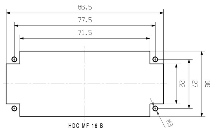
wycięcie montażowe
