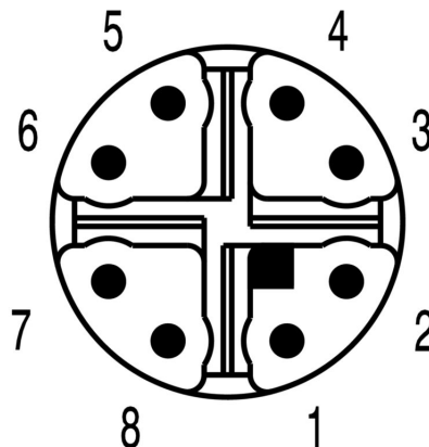
Schemat biegunów
