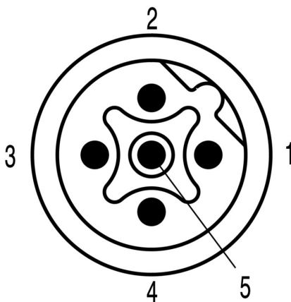
Schemat biegunów
