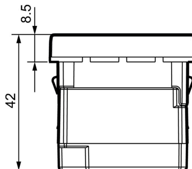
Rysunek wymiarowy
