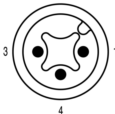
Schemat połączeń
