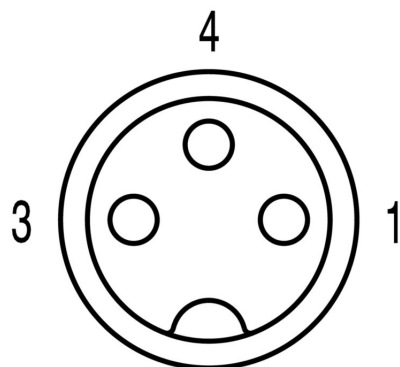
Schemat biegunów
