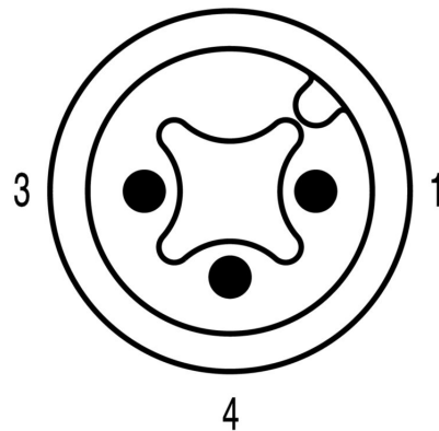
Schemat połączeń
