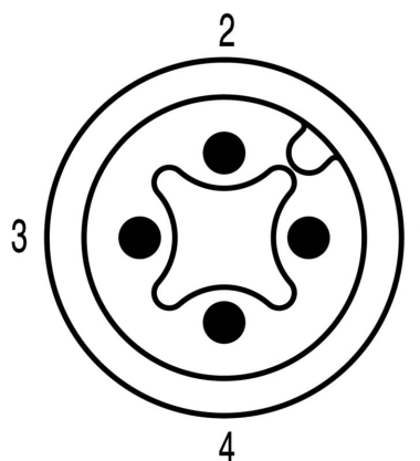
Schemat biegunów
