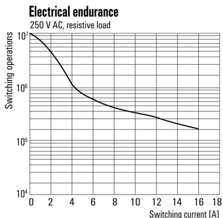
Trwałość elementów elektrycznych Obciążenie rezystancyjne
