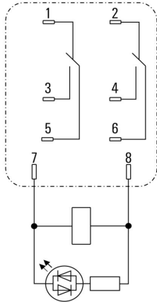
Widok kołków od spodu
