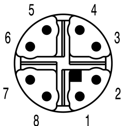
Schemat biegunów
