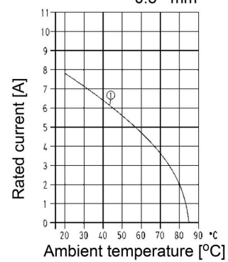
Krzywa obciążalności prądowej
