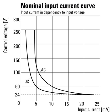
Prąd wejściowy w zależności od napięcia wejściowego
