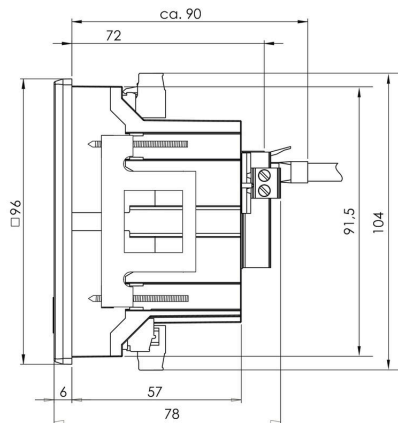
Rysunek wymiarowy
