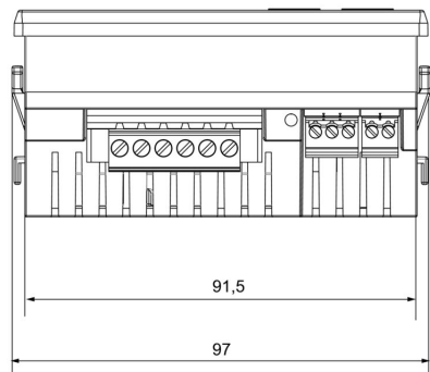
Rysunek wymiarowy
