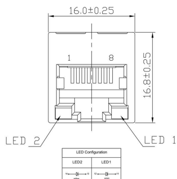
Rysunek wymiarowy
