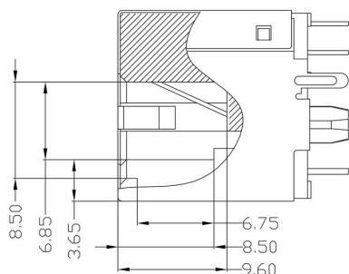
Rysunek wymiarowy
