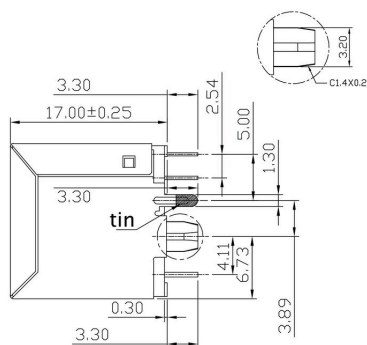
Rysunek wymiarowy
