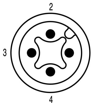
Schemat biegunów
