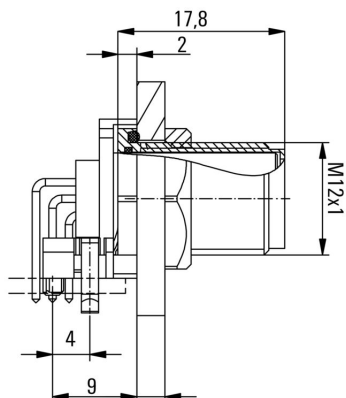
Rysunek wymiarowy
