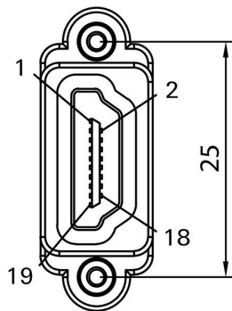
Rysunek wymiarowy
