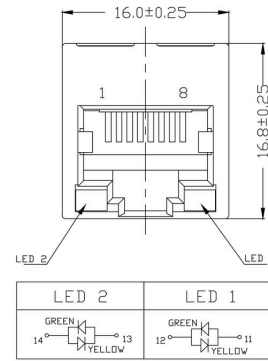
Rysunek wymiarowy
