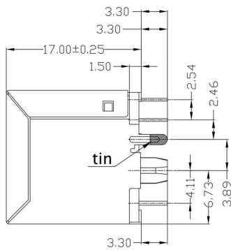
Rysunek wymiarowy
