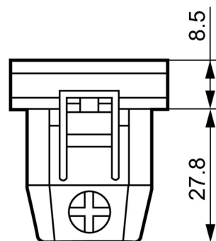
Rysunek wymiarowy
