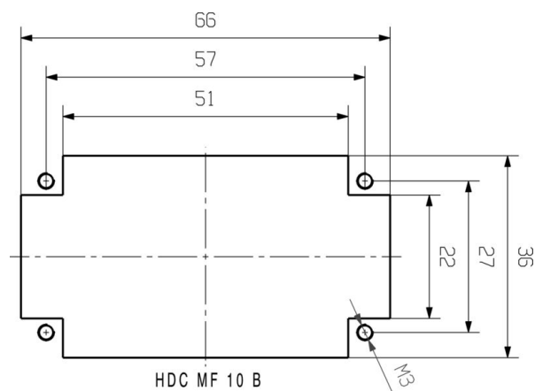
wycięcie montażowe
