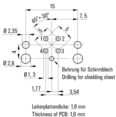
Schemat otworów wierconych
