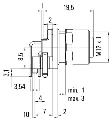
Rysunek wymiarowy
