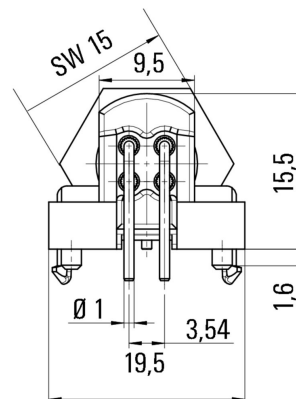
Rysunek wymiarowy
