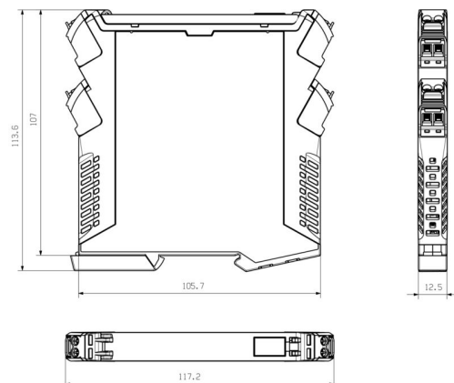
Rysunek wymiarowy
