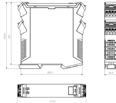
Rysunek wymiarowy
