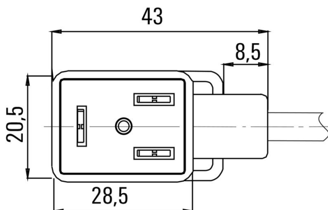
Schemat biegunów
