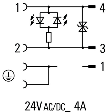
Schemat połączeń
