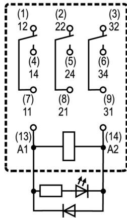
핀의 밀면도
