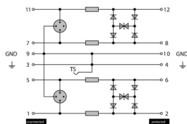
Complete module direct grounding, with remote signalling Komplettrmodul direkte Erdung, mit Fernmeldung
