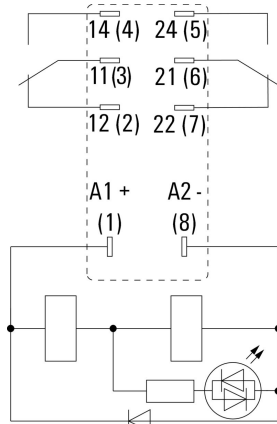
핀의 밑면도
