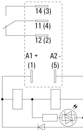
핀의 밑면도
