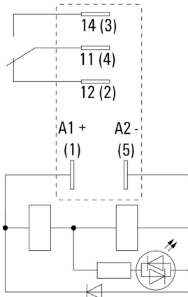
핀의 밀면도
