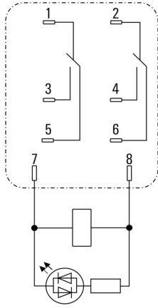
핀의 밑면도
