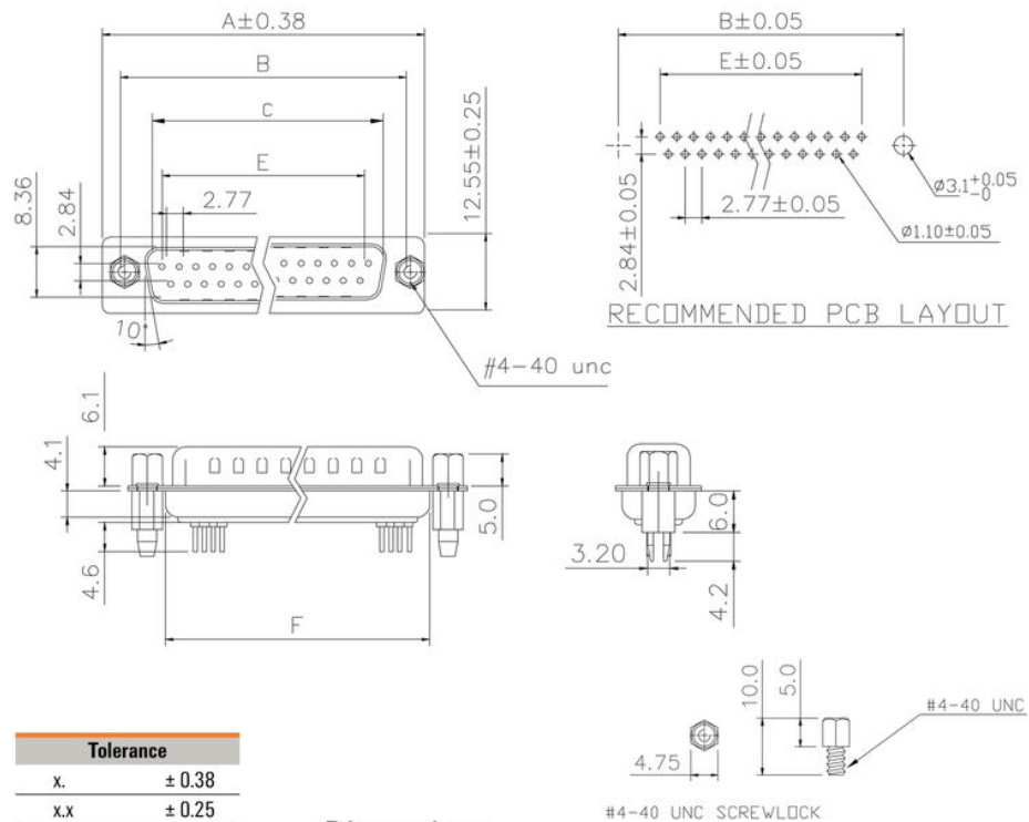
Dimensions
