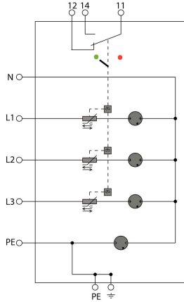
Prinzipschaltbild
