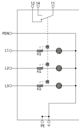
Prinzipschaltbild
