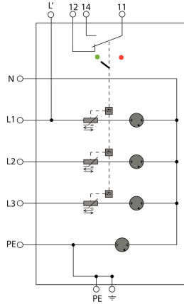
Prinzipschaltbild
