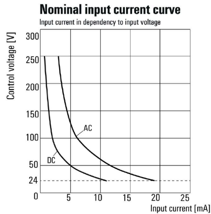
입력 전류에 대한 의존성이 있는 입력 전압
