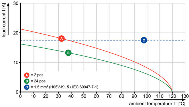
BLF 3.50/./180 - SL-SMT 3.50/./180
