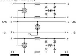
Complete module indirect grounding, with remote signalling Komplettrnodule indirekte Erdung, mit Fernmeldung
