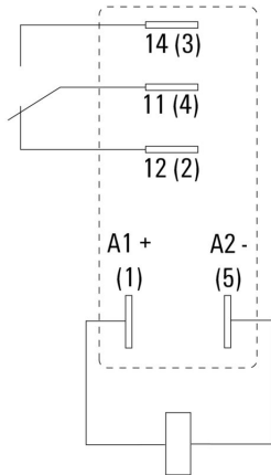
下からのピンのビュー
