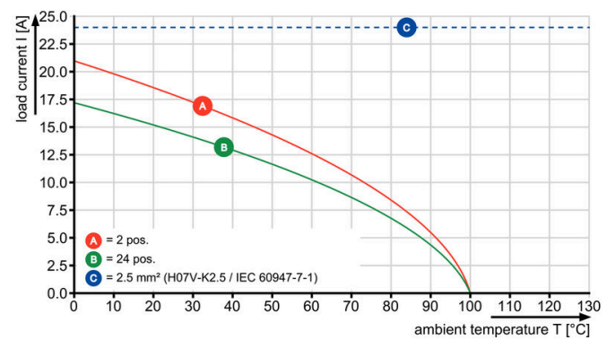
BLZP 5.08/.. /180 - SL 5.08/.. /90
