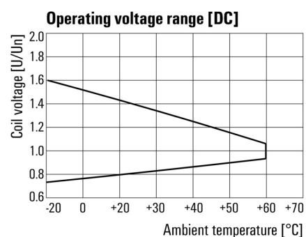
DC 動作電圧範囲
