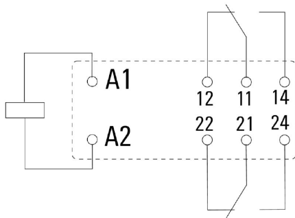
Vista dei pini dal basso
