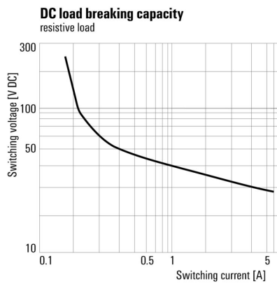
Curva limite di carico DC Carico ohmico
