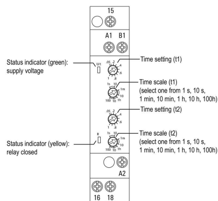
Disegno dettagliato
