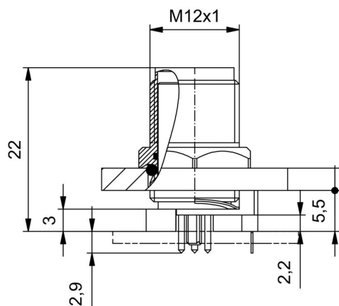
Disegno quotato
