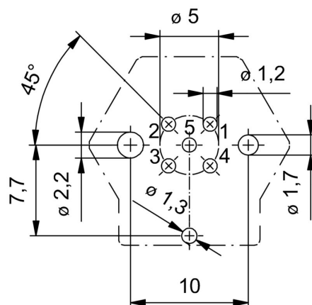
Disegno del circuito stampato
