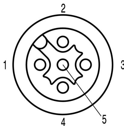
Schema dei poli
