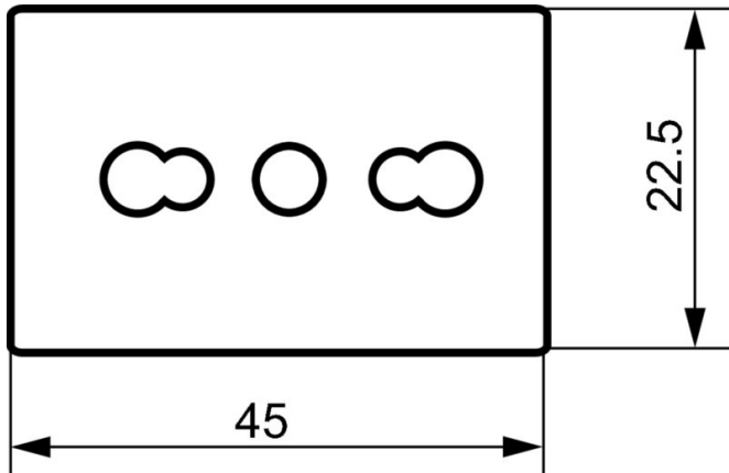
Disegno quotato
